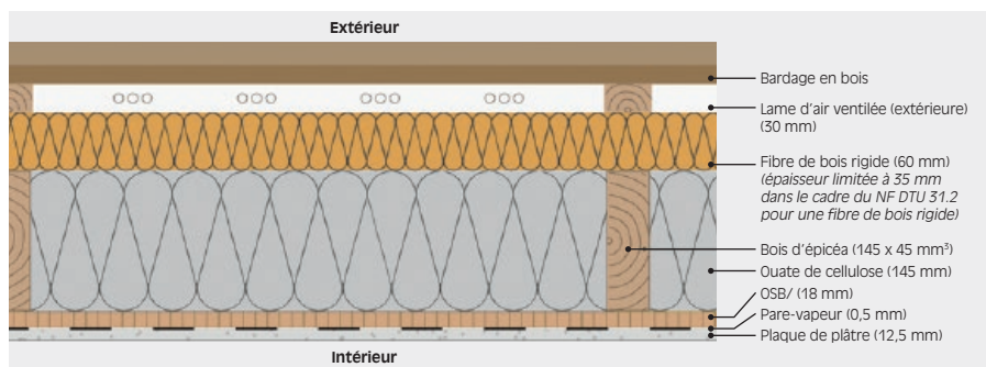
Mur à Ossature Bois avec ouate insufflée et pare-pluie en fibre de bois rigide. Déphasage : 11h50 Atténuation d'amplitude : 95%.
