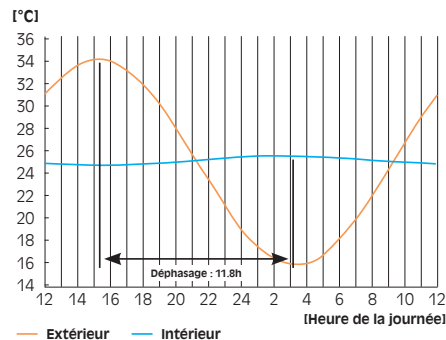
La courbe rouge présente l'évolution de la température d'une journée d'été. La courbe bleue présente le déphasage de l'onde de chaleur et la réduction de son amplitude.
